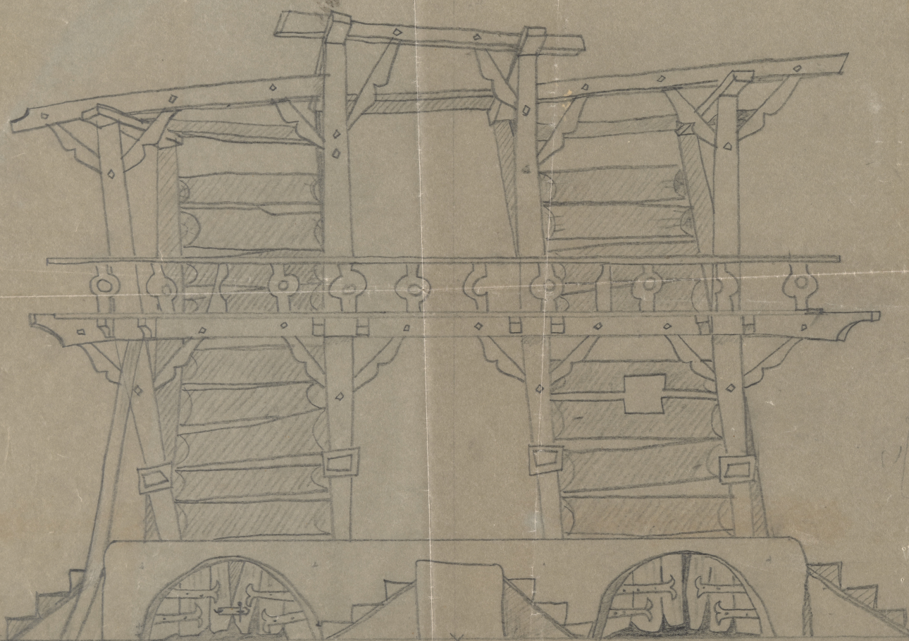
"ZYNIOT JOZEFA" WIDOK OBŁNY 1:25
